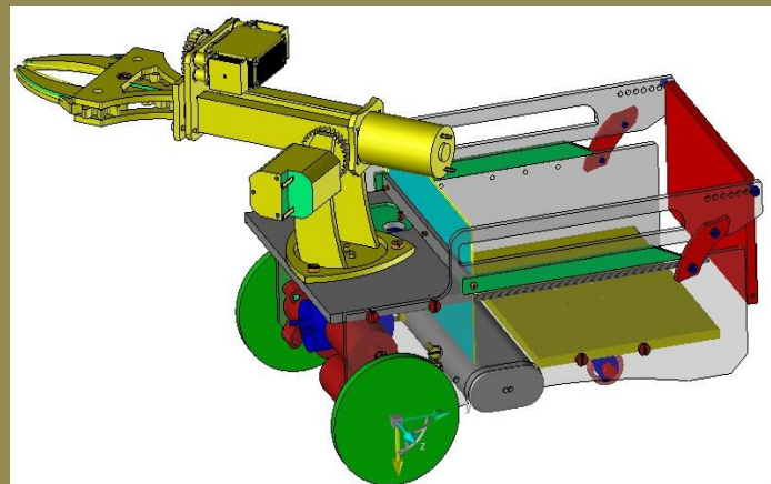
Τριδιάστατο μοντέλο του ROBOT
